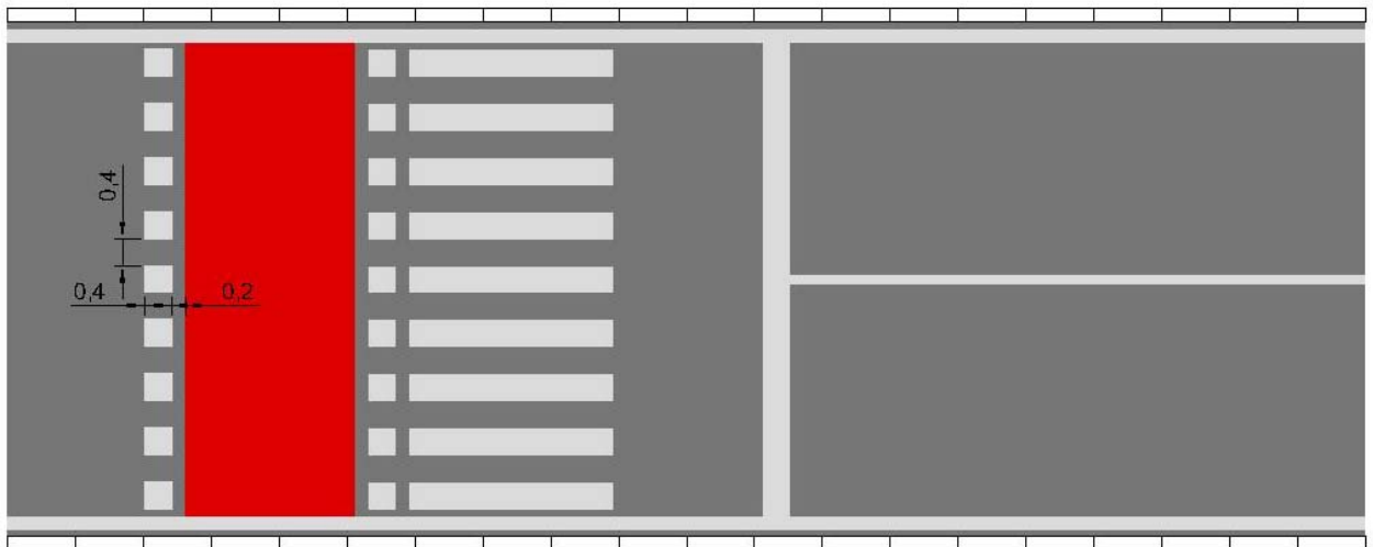
Figura 13 - Modelo de faixa de pedestre com travessia de ciclovia
