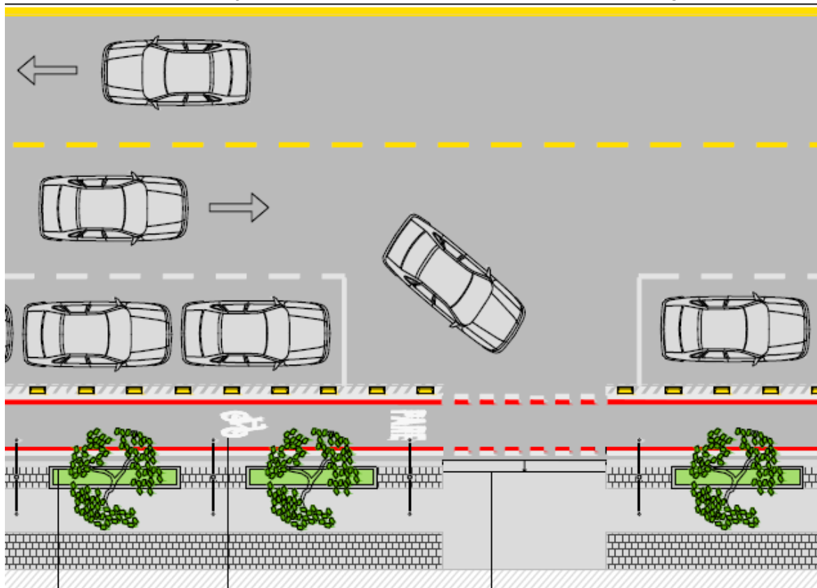
Figura 15 - Modelo de travessia de ciclista em entrada de lote
