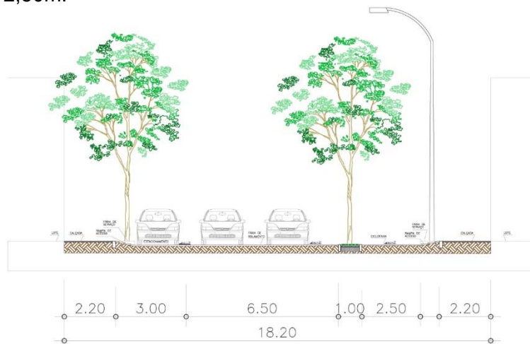
Figura 7 - Seção esquemática das Ruas 07, 10, 11 e 14
