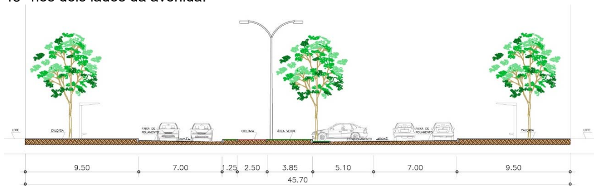
Figura 6 – Seção da Avenida Central do Centro Urbano. Estaca 14, Av. Central 03 e 04
