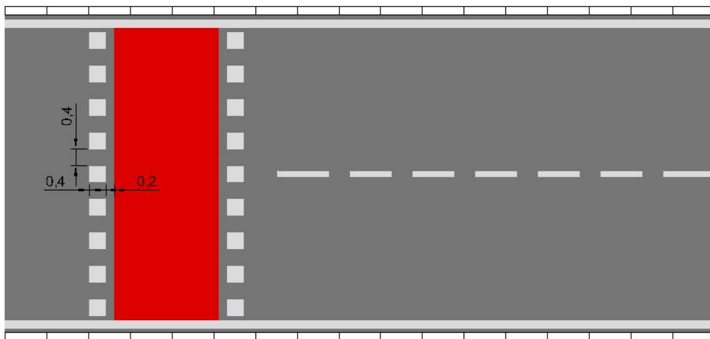
Figura 14 - Modelo travessia de ciclista sem faixa de pedestre
