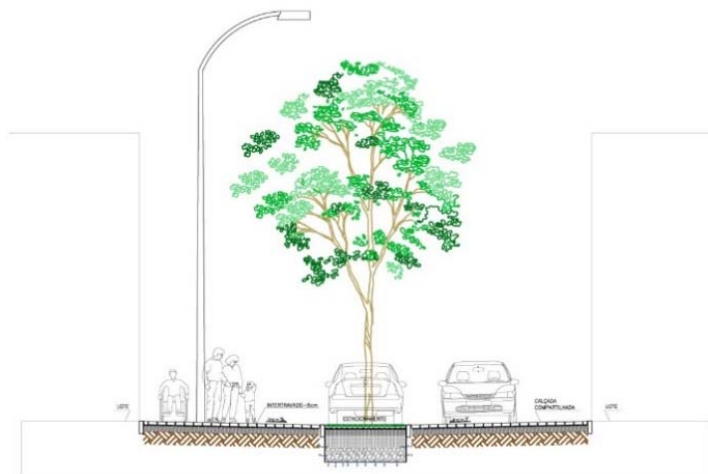
Figura 4 - Corte esquemático da rua compartilhada Ruas 5, 8, 13 e 15 e o caimento central
