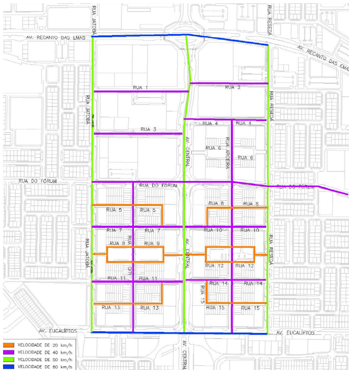
Figura 9 - Hierarquia e velocidade das vias
